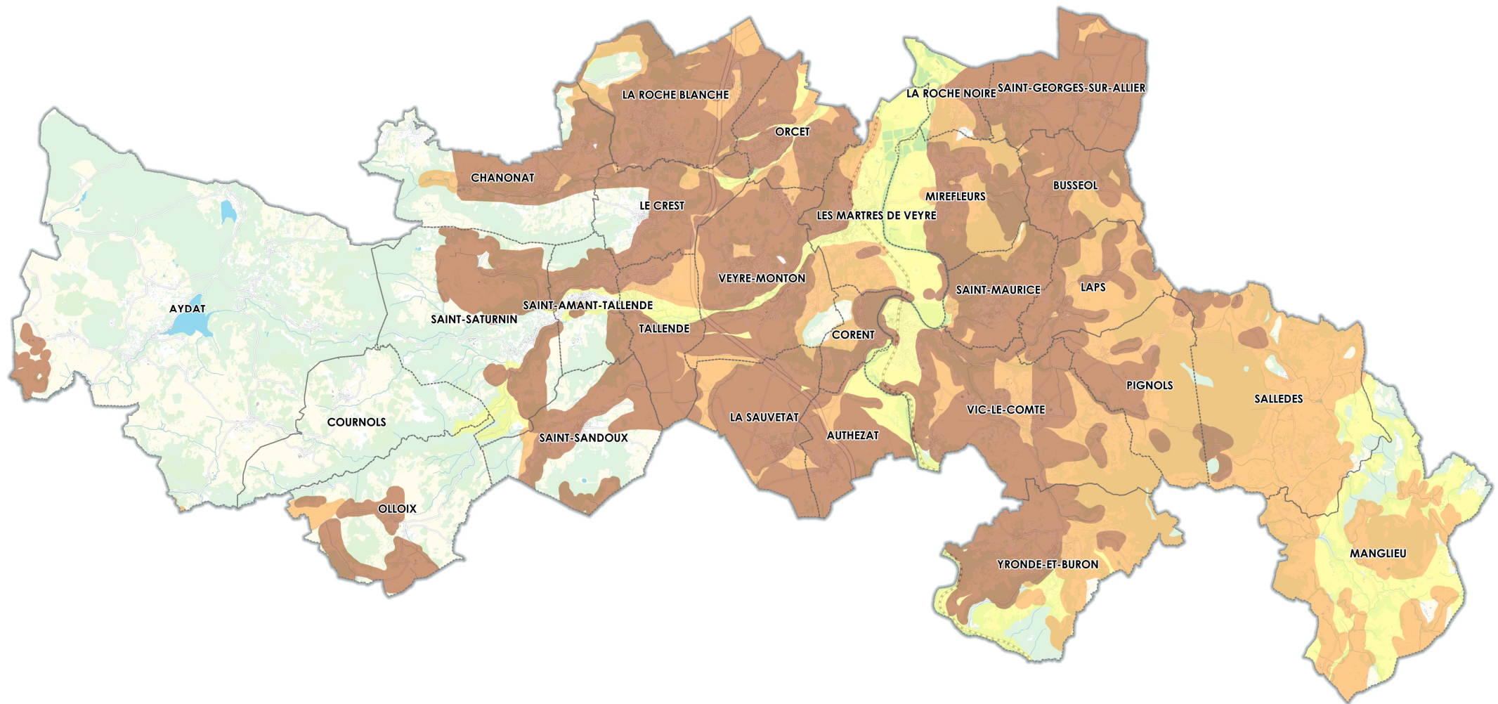
Aléa retrait-gonflements des argiles
